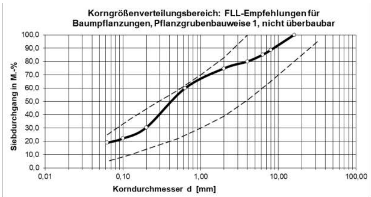
Bild 1: Korngrößenverteilung Baumsubstrat 0/16, Bezeichnung FLL 1 – Substrat mit empfohlenem Korngrößenverteilungsbereich für ein nicht überbaubares Baumsubstrat gemäß FLL
